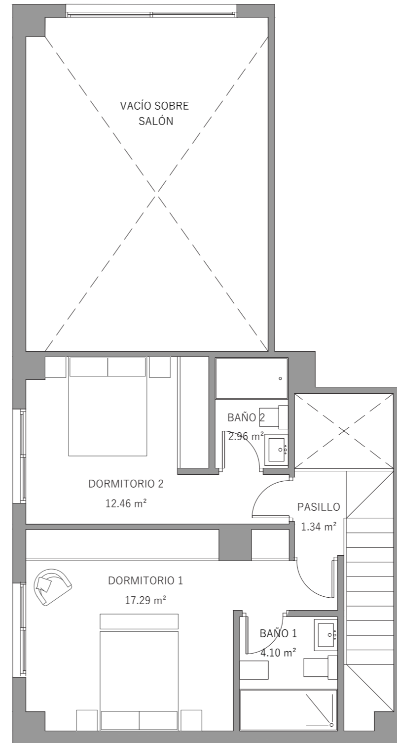
ENTREPLANTA
